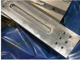
Einsätze-Prägewerkzeug
