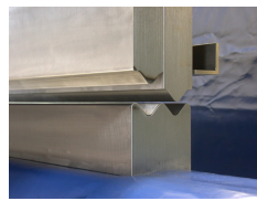
fertiges Wellenprofil
