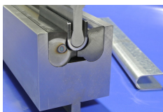
U-Bieger mit beschichteten Backen, gegen Zinkabrieb
